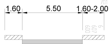
presjek 10-10
