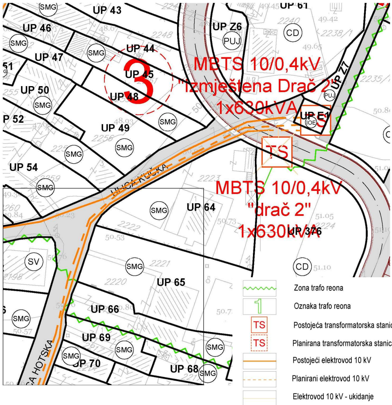
Izvod iz grafičkog priloga Detaljnog urbanističkog plana "Drač – putnički terminal"
