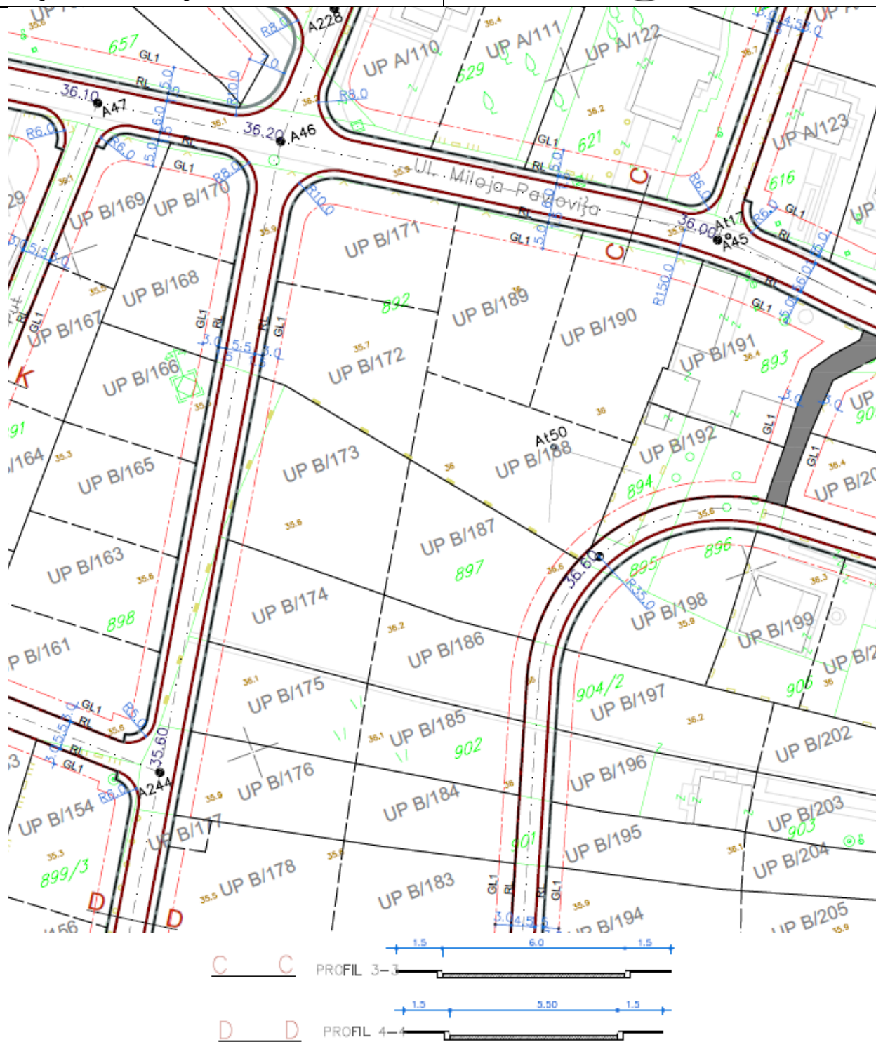
GRAFIČKI PRILOG – Plan saobraćajne infrastrukture Izvod iz DUP-a "Gornja Gorica 1" u Podgorici za urbanističku parcelu B 173 u zoni B
