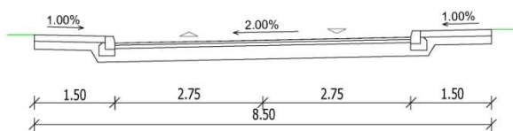
presjek D - D
