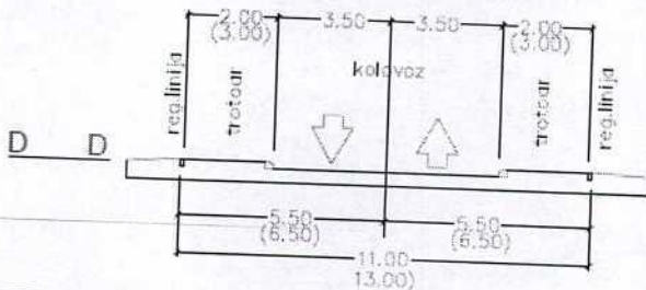
GRAFIČKI PRILOG – Plan saobraćaja, nivelacije i regulacije
