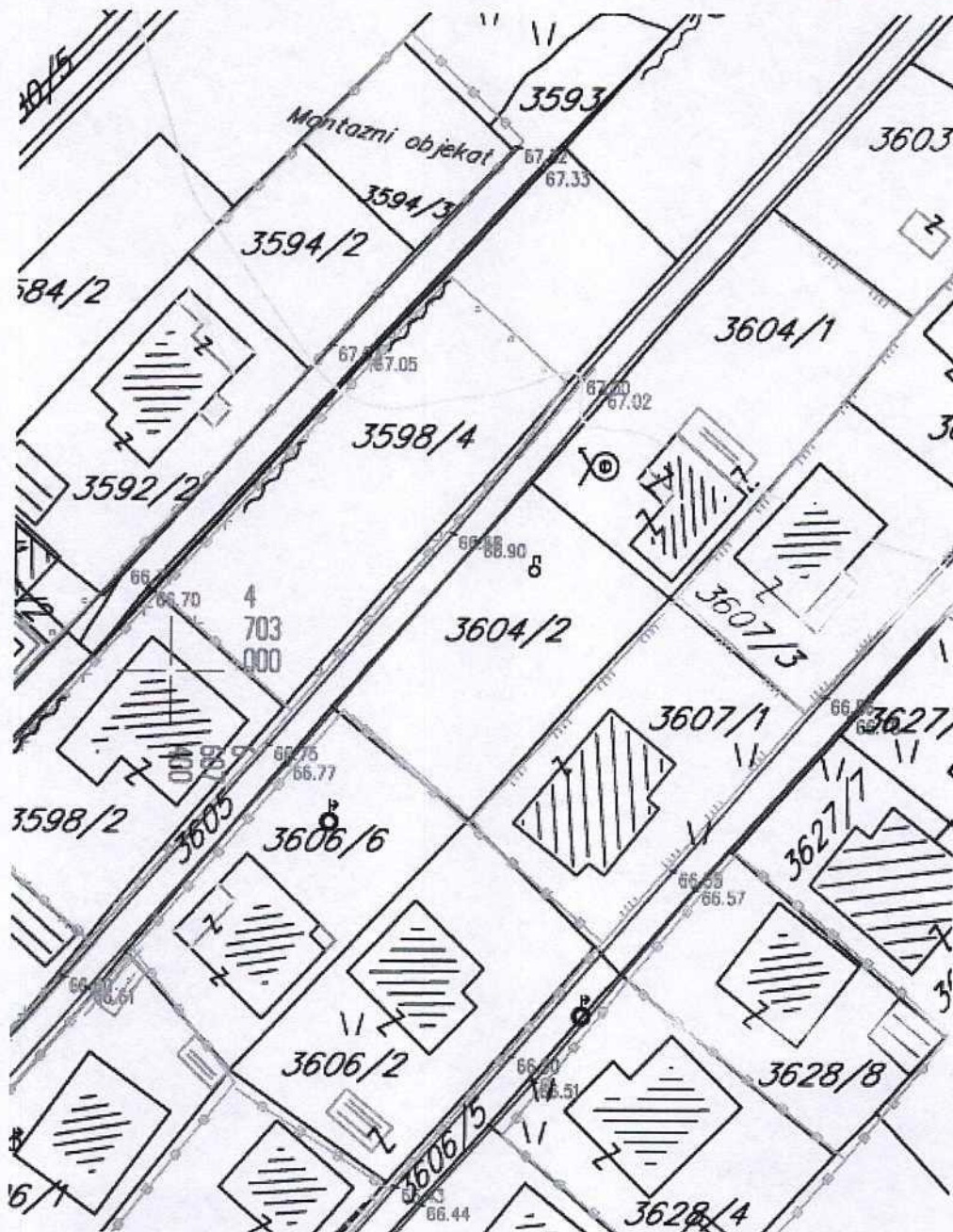
GRAFIČKI PRILOG – 1.2 Topografsko katastarska podloga sa granicom zahvata Izvod iz DUP-a "Murtovina" za urbanističku parcelu UP 436, zona C
