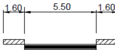
presjek 3-3
