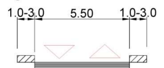
presjek 30-30
