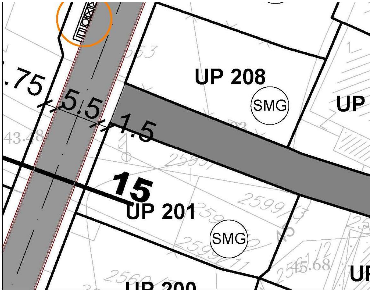
presjek 15-15
