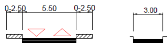
presjek 2 - 2 presjek 8 - 8
