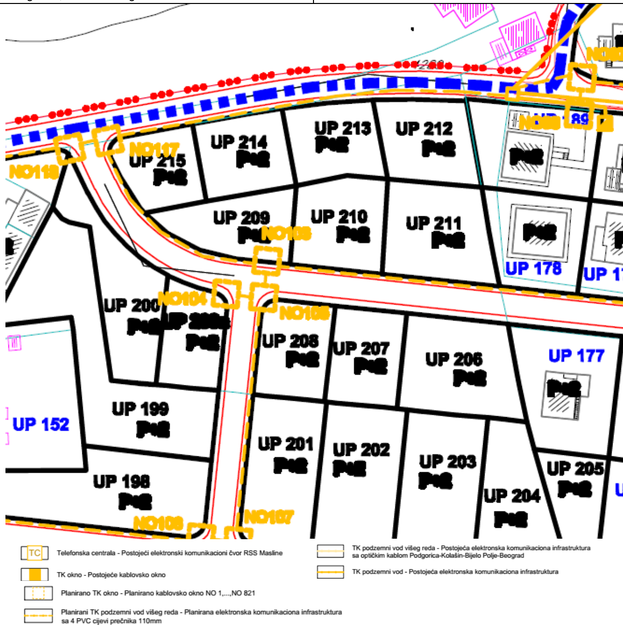
GRAFIČKI PRILOG – Plan elektronska infrastruktura Izvod iz DUP-a "Zlatica B" u Podgorici za urbanističku parcelu UP213 u zoni A
