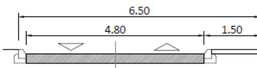
PRESJEK 7-7 (Ulica Tivatska, Ulica 1, Ulica 2, Ulica 3, Ulica 4, Ulica 6, Ulica 8, Ulica 9, Ulica 12, Ulica 13,)
